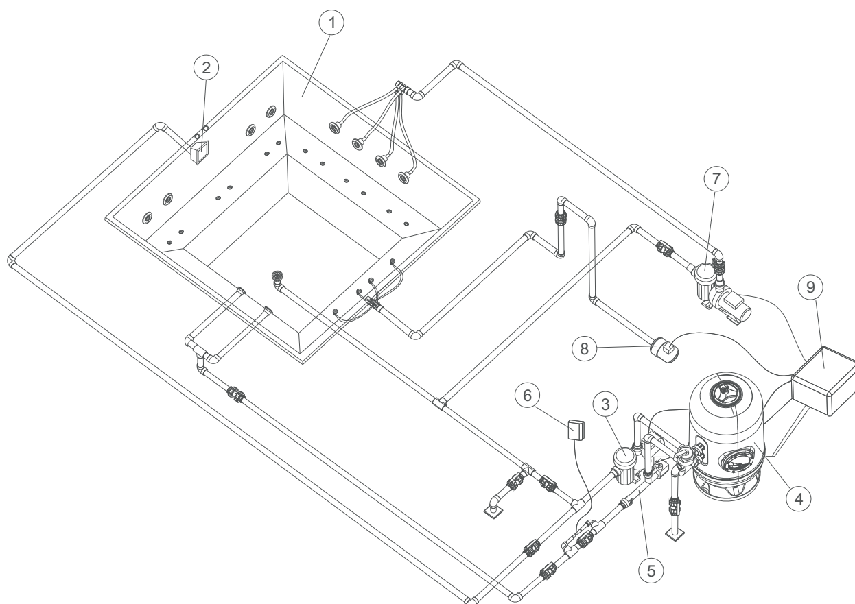
Esquema geral Spa com Skimmer
