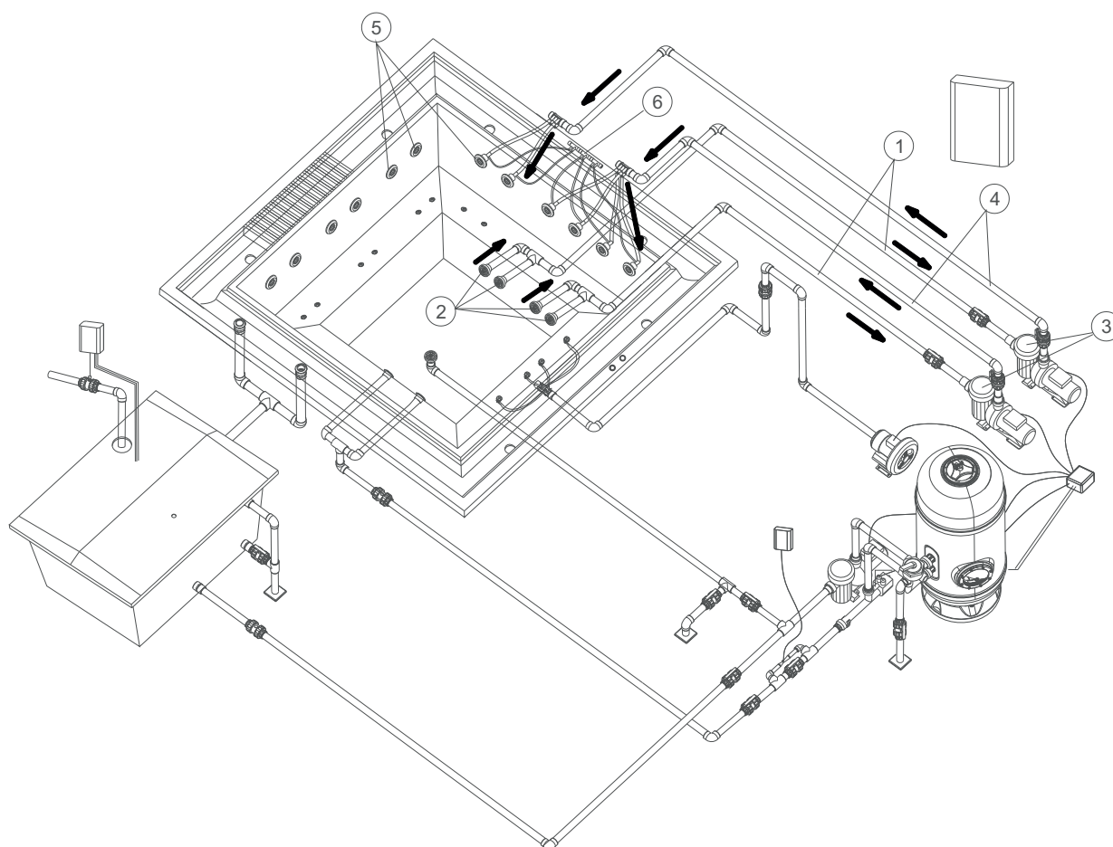
Esquema Massagem Água Spa.
