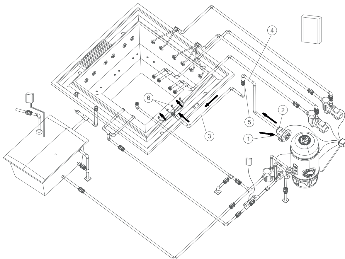
Fig. 1 Esquema Massagem Ar Spa.
