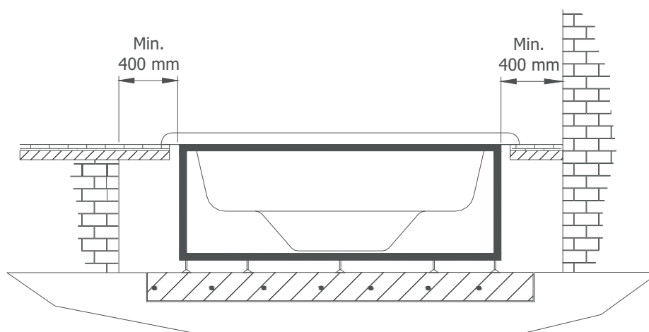
Esquema Distância mínima à volta do Spa.
