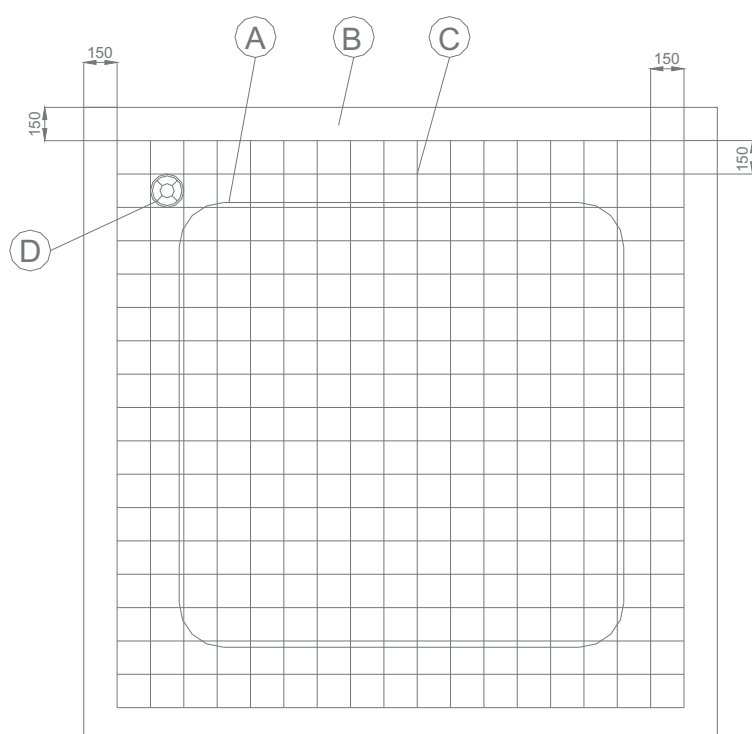
Esquema Cimentação.
