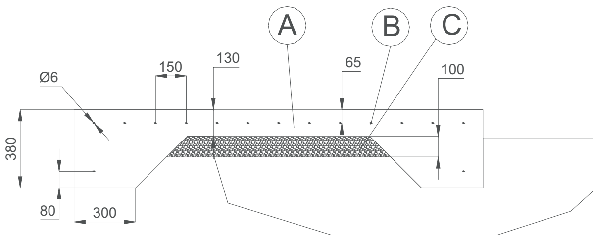
A: Lajes de cimento B: Varetas de aço C: Areia compactada Todas as dimensões em mm.
