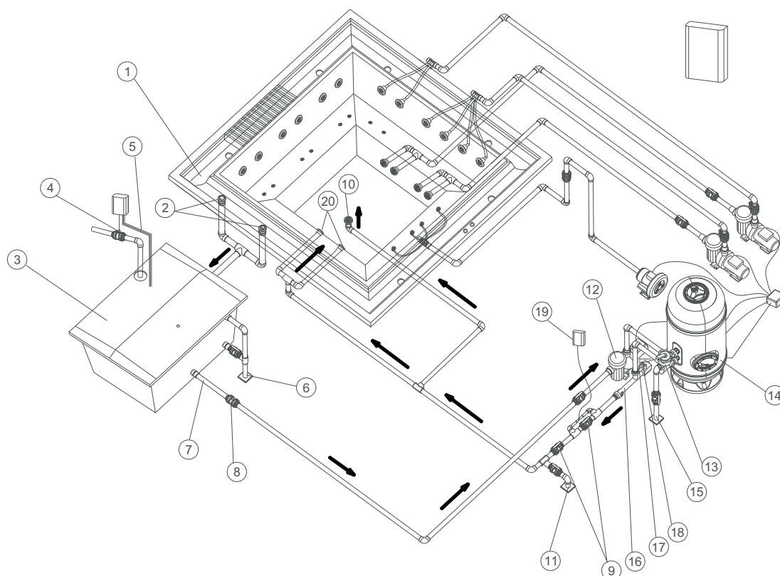
Esquema recirculação Spa com Transbordante Opção B.
